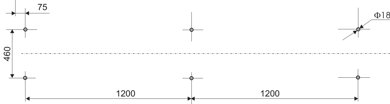
RASPORED OTVORA U POSTOLJU ZA VEZU SA FUNDAMENTOM
